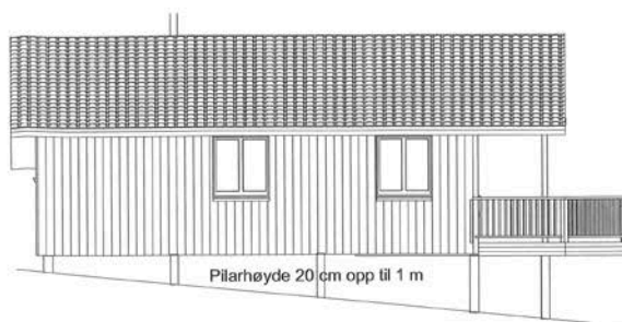
Fasade vest
