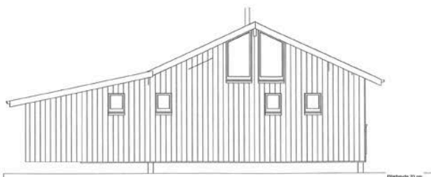
Fasade nord
