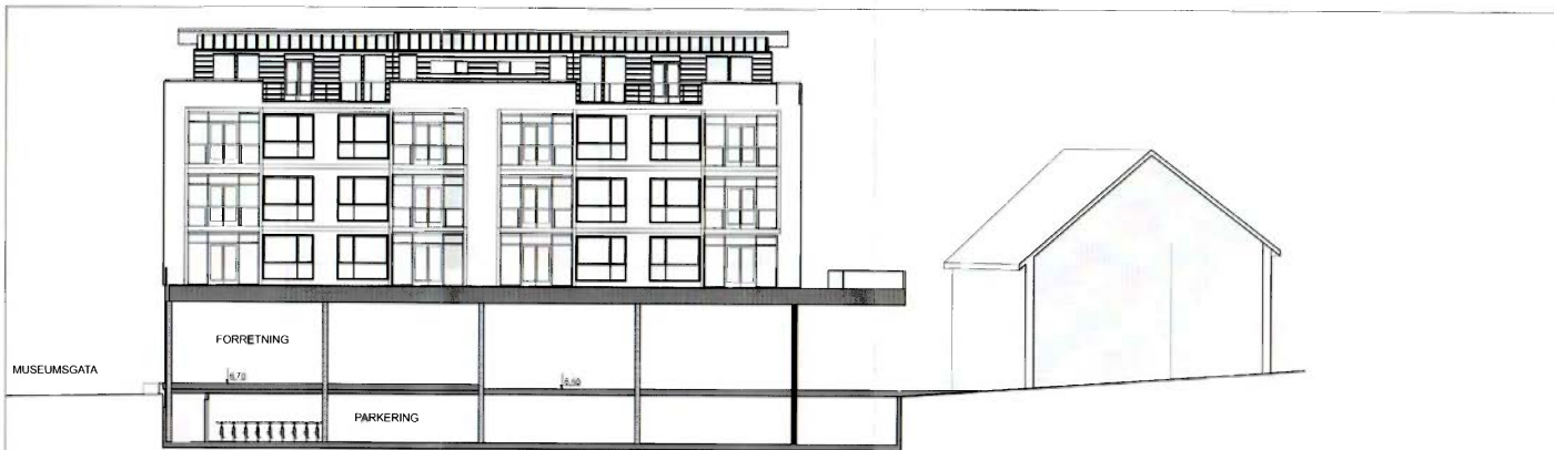
FASADE SØR - BYGG 2 1 : 200
