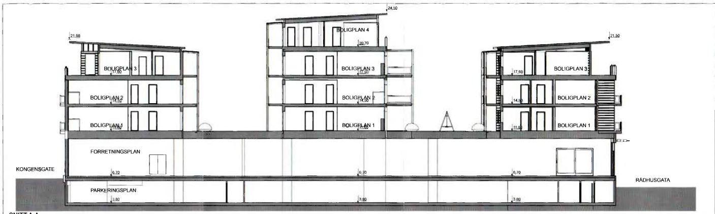
SNITT A-A 1 : 200
