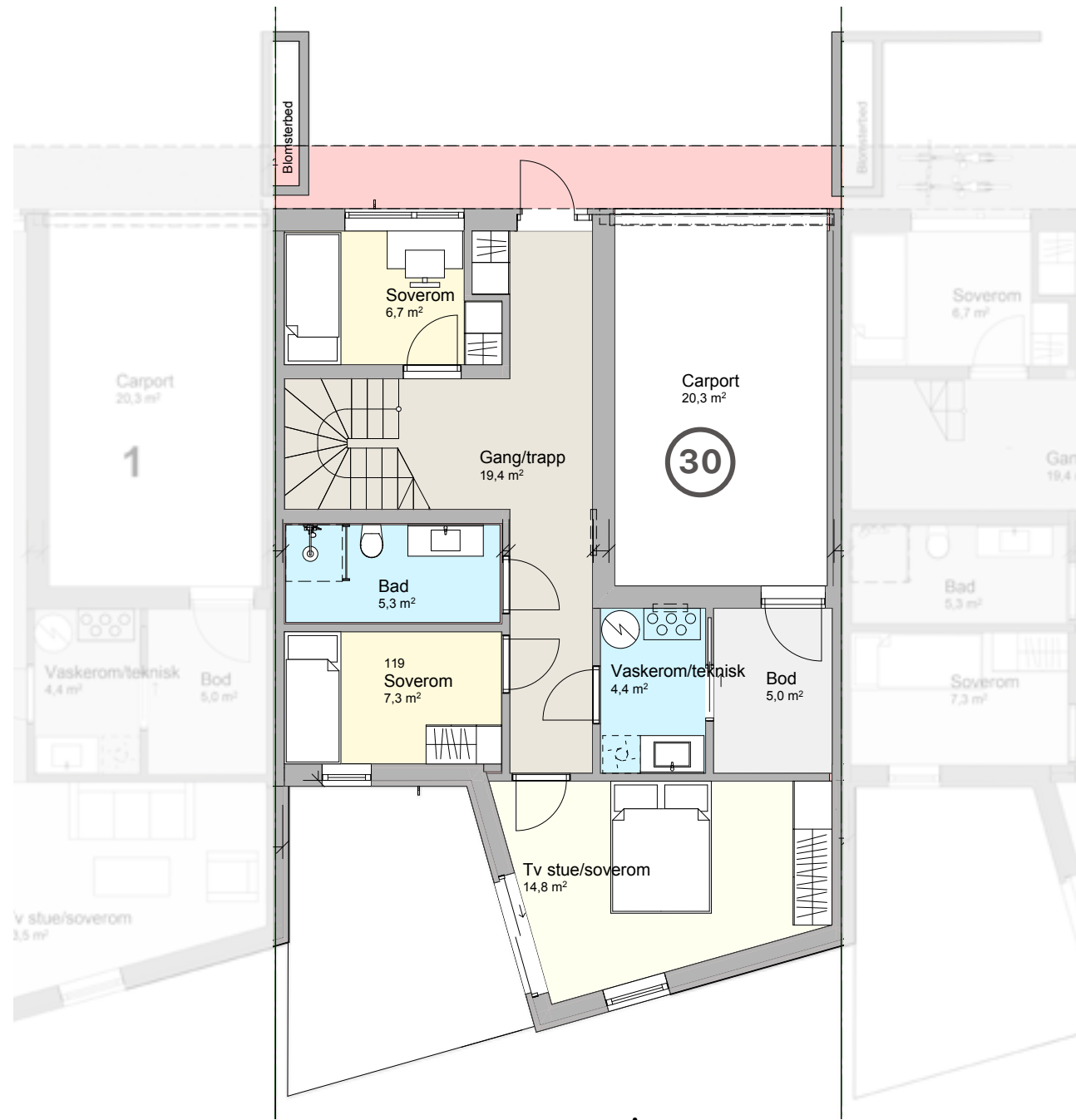
Første etasje
