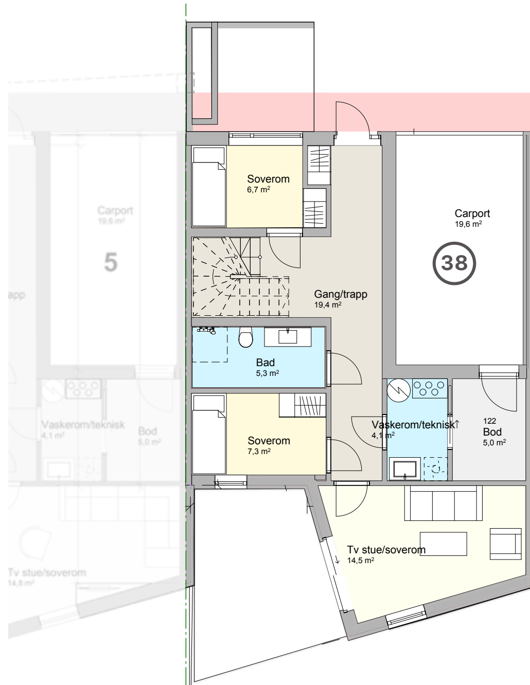
Første etasje
