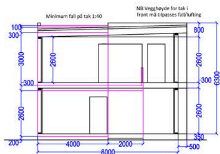
Prestekragveien 19- Snitt C-C
