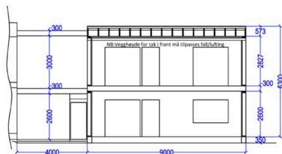
Prestekragveien 21-25- Snitt B-B
