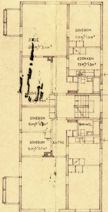
2. ETASJE
