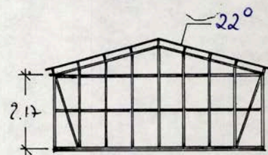
SNITT
