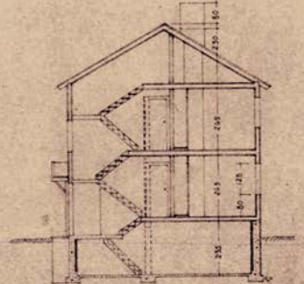
SNITT
