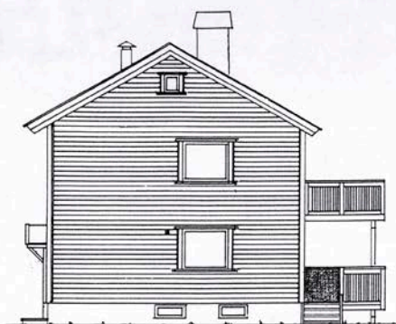
FASADE MOT VEST
