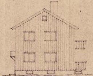
NORD.
