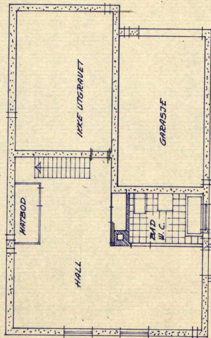
UTBEDRET UNDERETASJE
