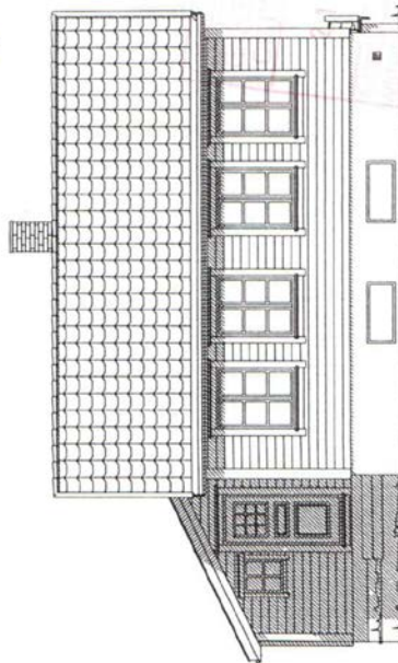
Fasade vest
