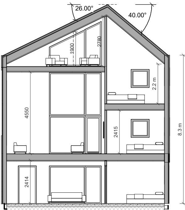
Snitt
