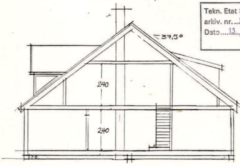
SNITT
