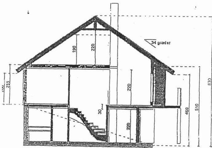
TVERRSNITT MIDTSEKSJON
