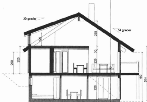
Snitt gjennom hems i midtseksjon.
