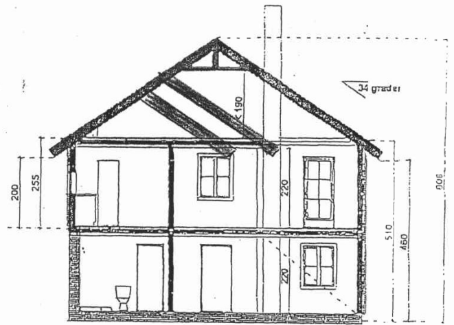
TVERRSNITT ENDESEKSJON
