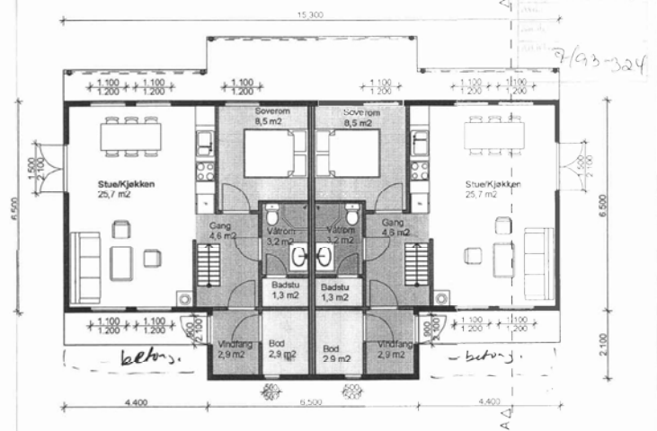
Plan hovedetasje
