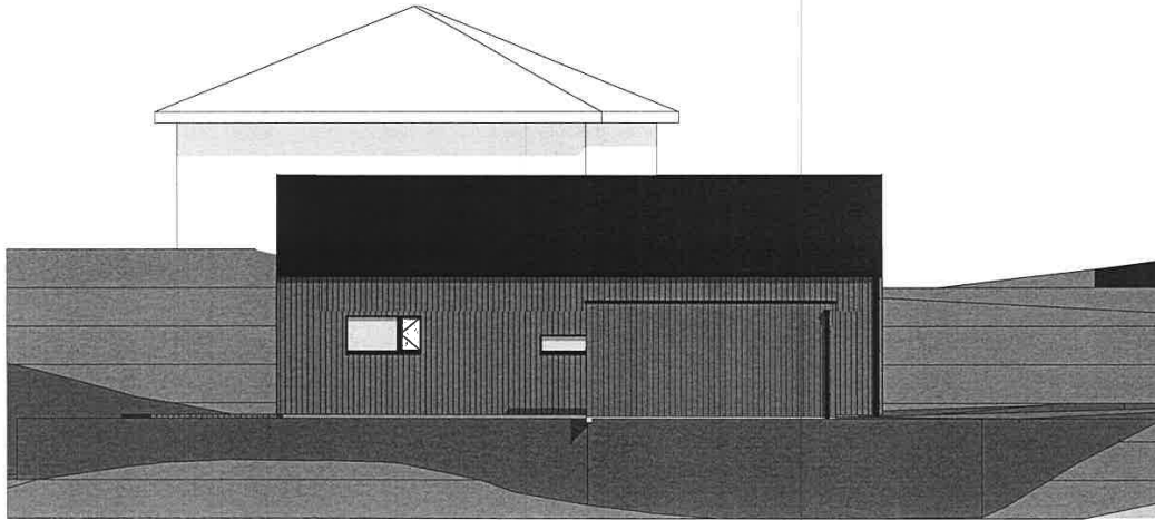
1:100 Fasade Sør
