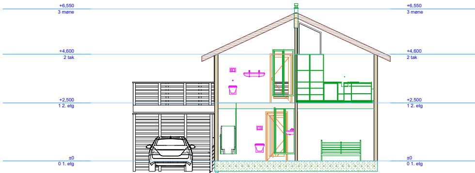
Snitt sør (3)
