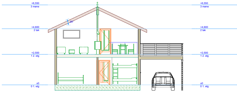
Snitt nord (2)
