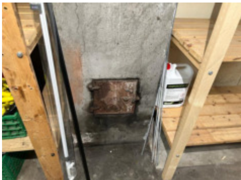
Sprekk i pipestamme, rust på sotluke, merker etter sotvann
