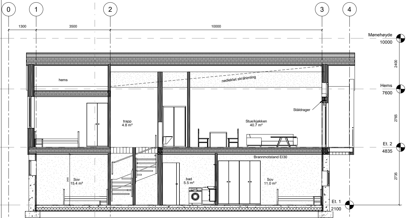
Snitt B-B 1 : 50
