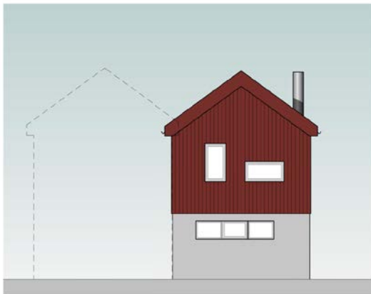
Øst 1 : 100
