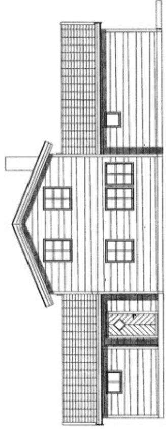
FASADE MOT: VEST
